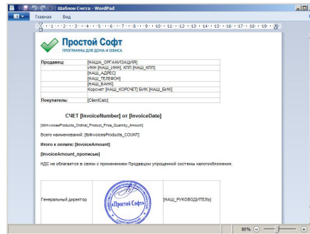
RTF-шаблон
