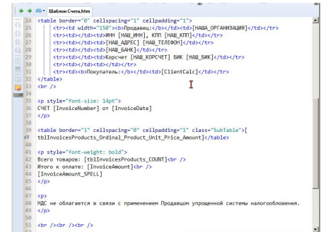
HTML-шаблон
