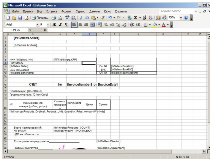
Excel-шаблон
